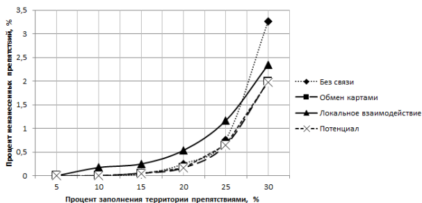
Рис. 7. Средний процент не нанесенных препятствий для разных методов.
