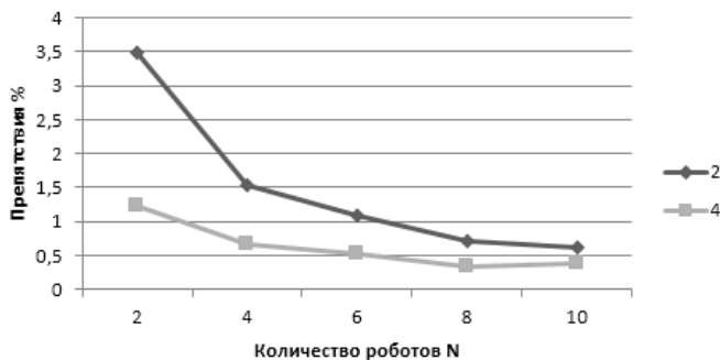
Рис. 5. Средний процент обнаруженных препятствий для лабораторного полигона.
