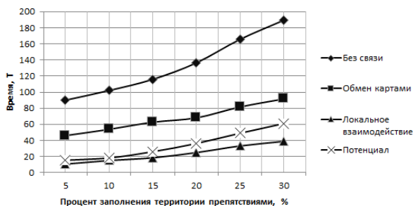
Рис. 8. Время исследования для разных методов.
