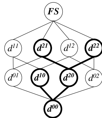
Рис.5. Диаграмма Хассе понятийной системы совместного функционирования агентов 1 и 2.
