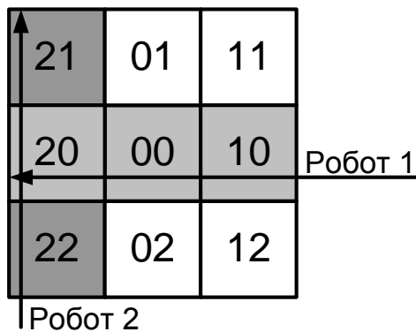
Рис.2. Подпространства классов состояний понятийной системы агентов 1 и 2.
