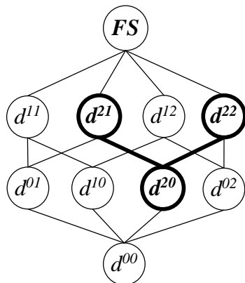
Рис.4. Диаграмма Хассе понятийной системы агента 2.
