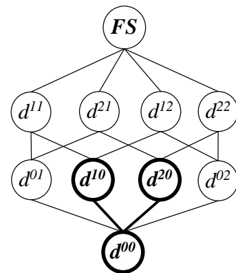
Рис.3. Диаграмма Хассе понятийной системы агента 1.
